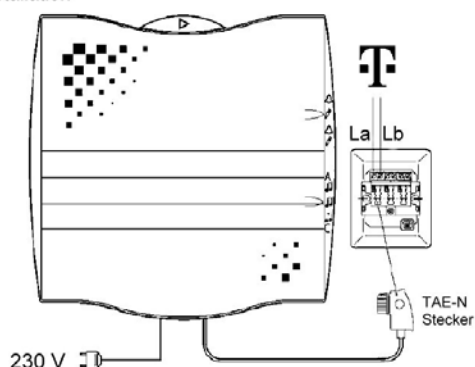
Aufputzinstallation
