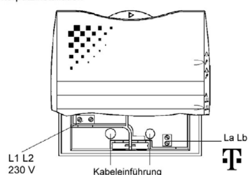
Unterputzinstallation
